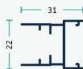
03 Guía de Retención
